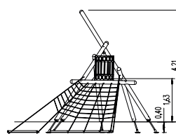
5 66 312 5 elbe tema Sand Wreck, Mast 1:200
